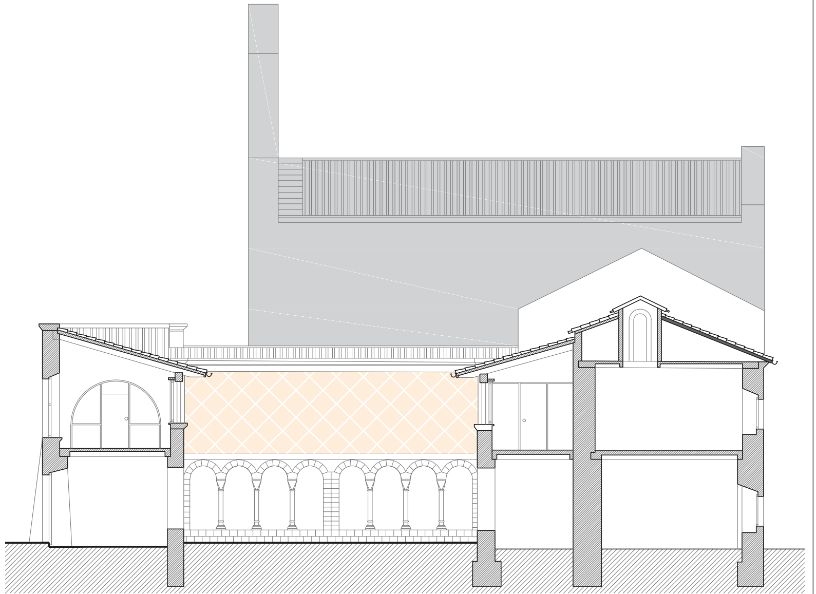
Sección A-A'
