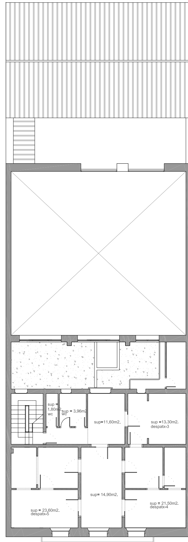
Primer pis
