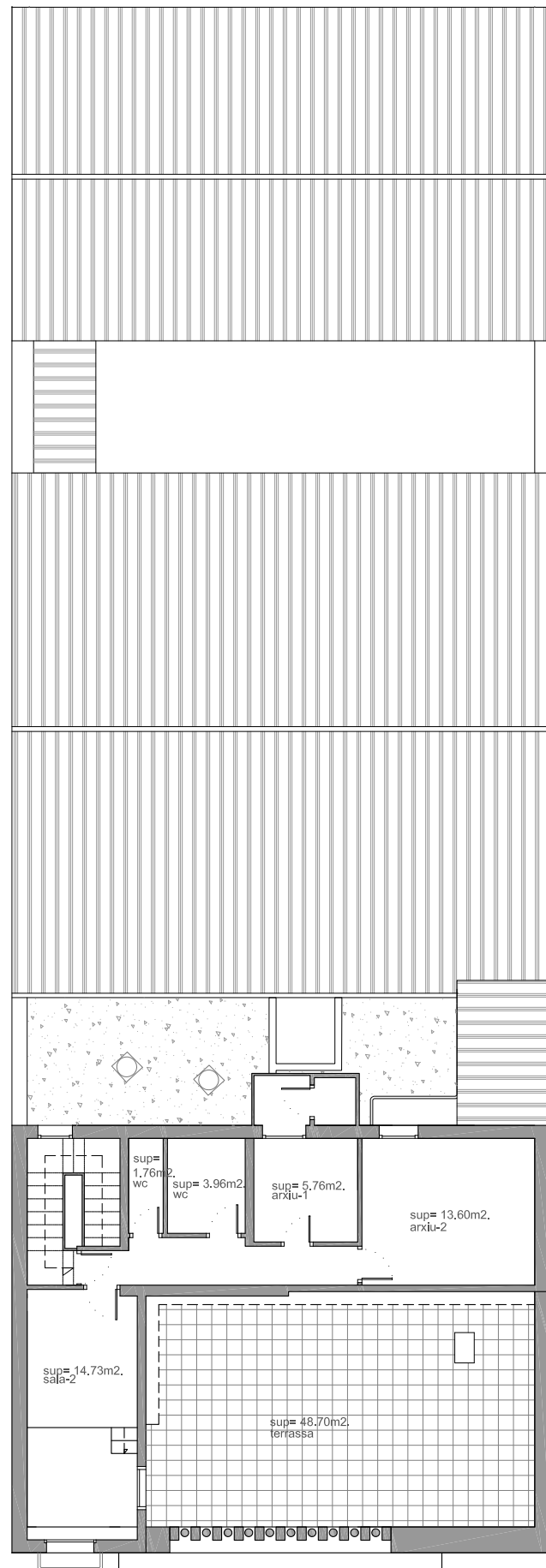
Segon pis
