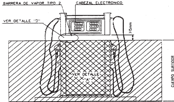
ALZADO
