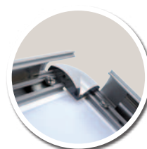
Apertura / cierra mediante perfil abatible
