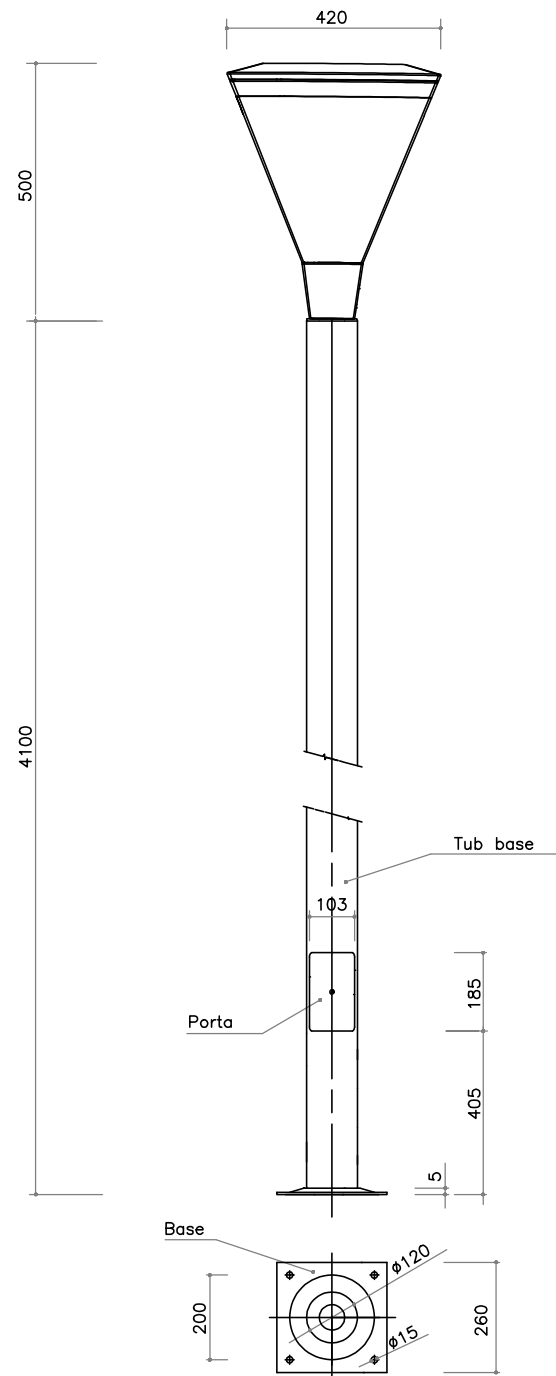
COLUMNA SERIE ROURA PLUS AMB LUMINARIA ELBA
