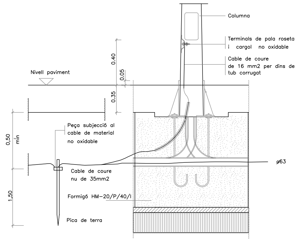
FONAMENT COLUMNA TIPUS I PICA DE TERRA ESCALA - / -
